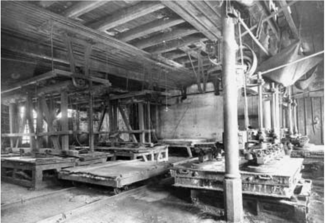
Abb. 1: Schleifapparat (rechts) und Stangenpoliere (links) in einem Schleif- und Polierwerk des 19. Jahrhunderts.
